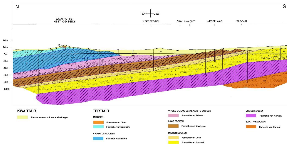
Fig. 3: Geologische Noord-Zuid doorsnede ter hoogte van Haacht.. De tertiaire afzettingen duiken naar het noorden. In het pleistoceen hebben de rivieren een brede geul uitgeschuurd die opgevuld is met dikke fluviatiele en eolische pakketten (Keijers 2014: 30)
