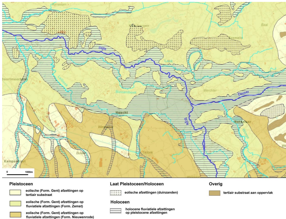
Fig. 2: De Pleistocene en Holocene afzettingen in de omgeving van Rotselaar, Werchter en Haacht (Bogemans, 2007)
