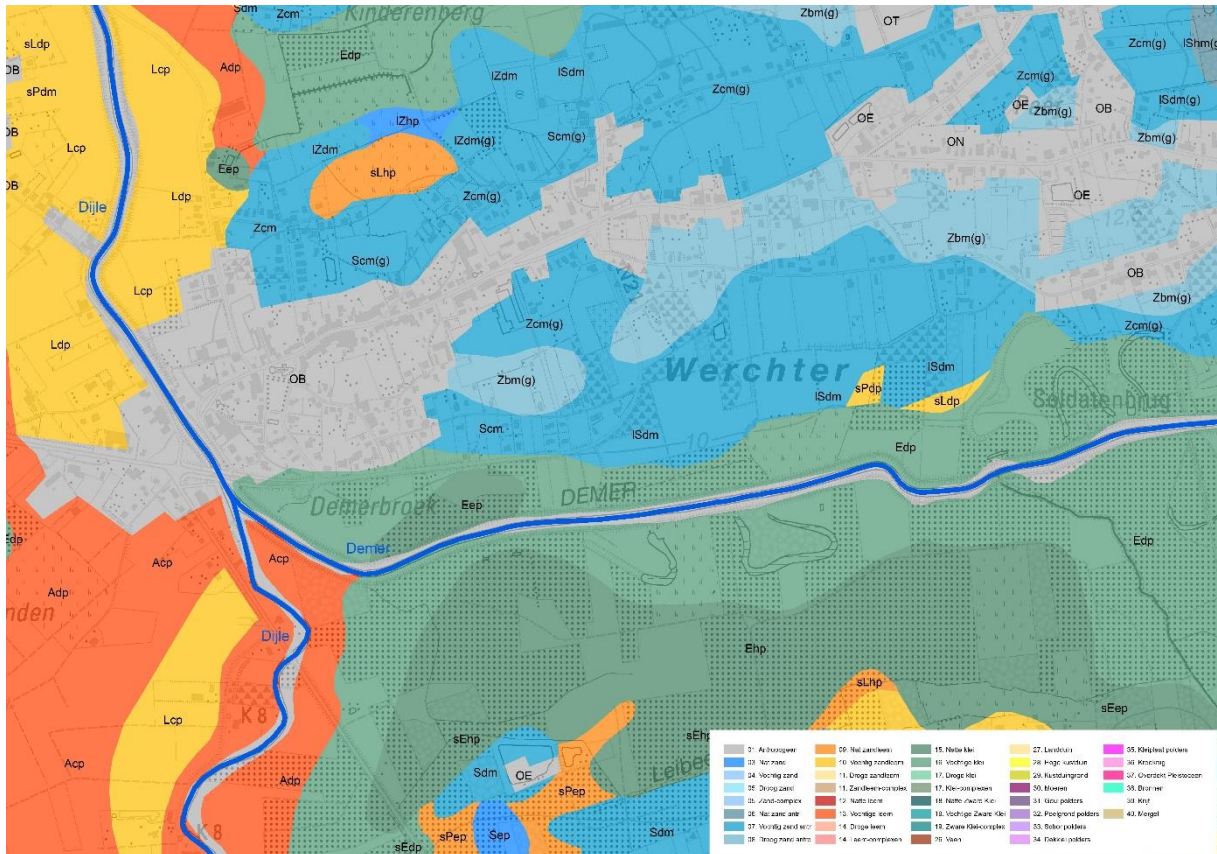
Fig. 5: Gecomprimeerde bodemkaart van omgeving Werchter waarbij de Holocene afzettingen de gele, rode en blauwe bodems zijn, waar de Pleistocene bodems samenvallen met de blauwe kleuren. De grijs ingetekende delen zijn door bewoning, groeve activiteiten, of sterke ophoging of vergraving niet gekarteerd kunnen worden (© AGIV)
