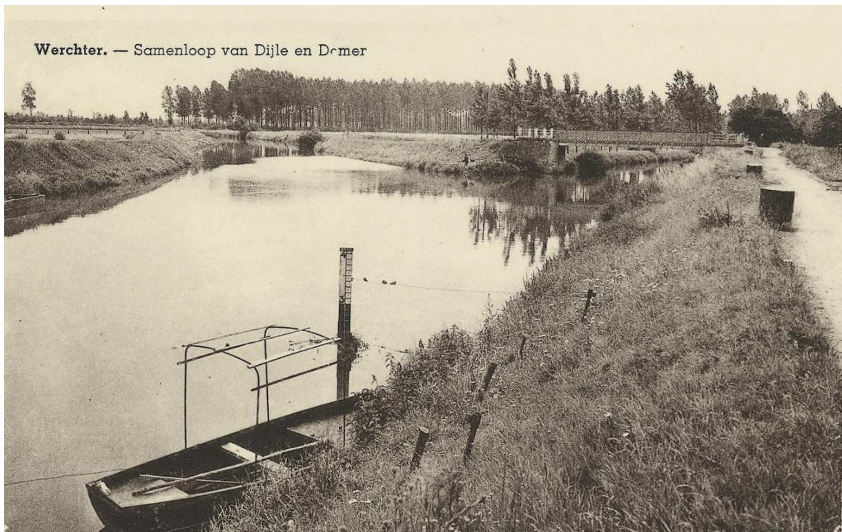
Fig. 113: De Demer-Dijle samenvloeiing rond de jaren 60 ( www.delcampe.net )
