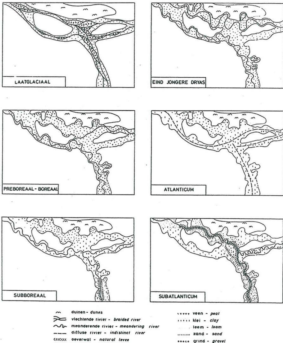
Fig. 4: Overzicht van de bewegingen van Demer en Dijle sinds de laatste IJstijd (De Smedt 1973: 123)
